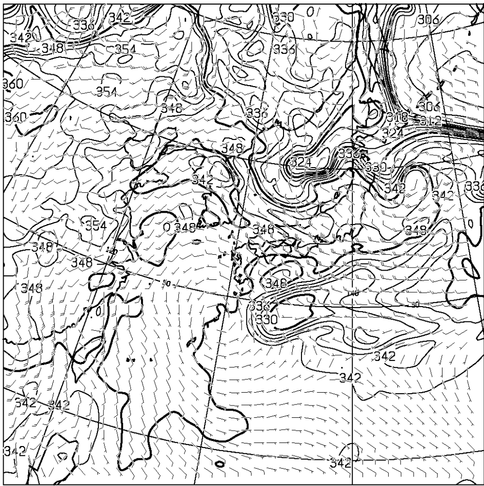
T=48 850hPa: E.P.TEMP(K),WIND(KNOTS) VALID 040000UTC
