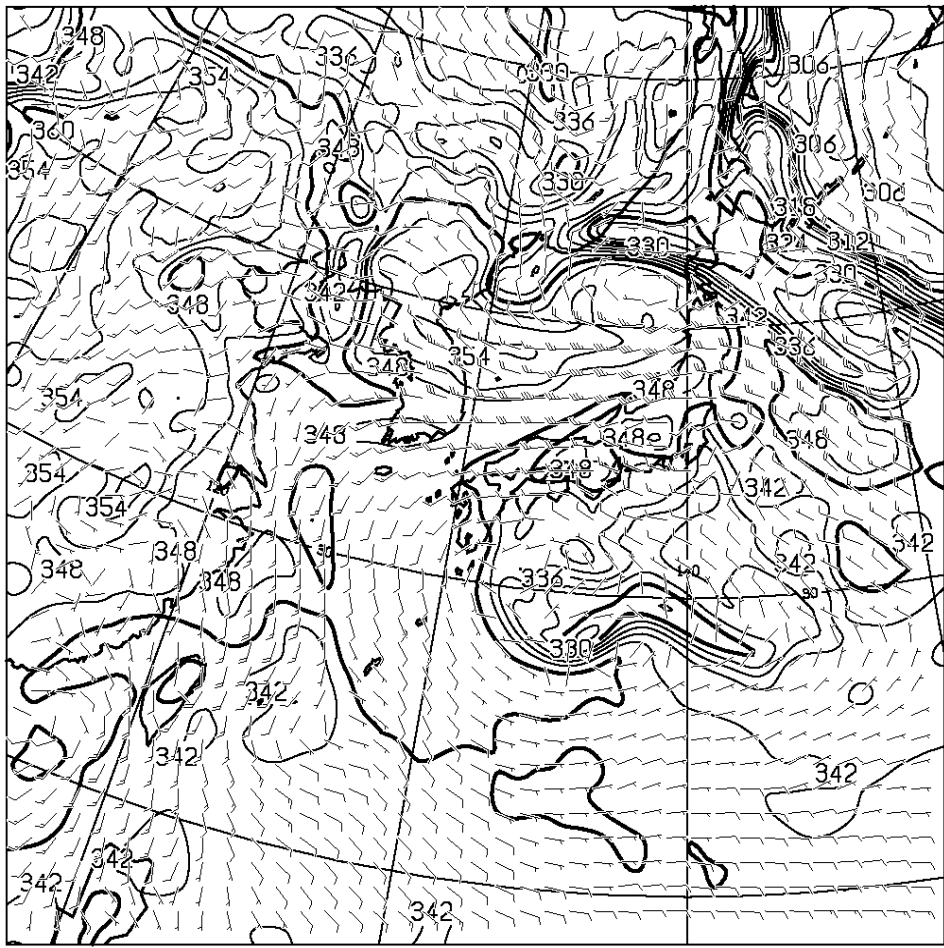
T=24 850hPa: E.P.TEMP(K),WIND(KNOTS) VALID 030000UTC
