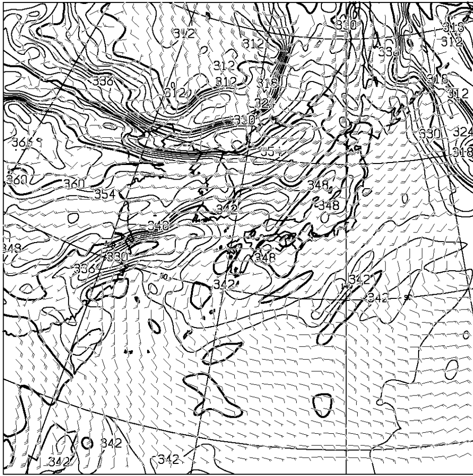
T=24 850hPa: E.P. TEMP(K), WIND(KNOTS) VALID 080000UTC
