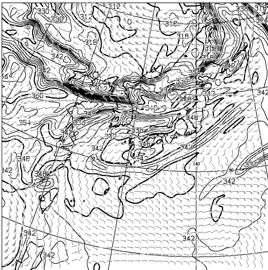
T=48 850hPa: E.P. TEMP(K), WIND(KNOTS) VALID 090000UTC
