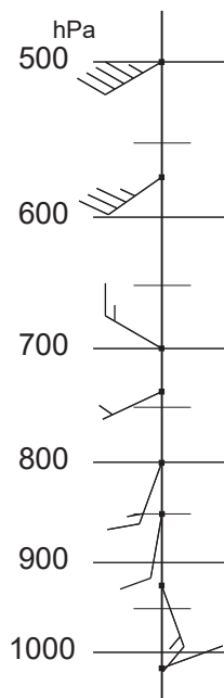
図 2 館野における風の鉛直プロファイル
