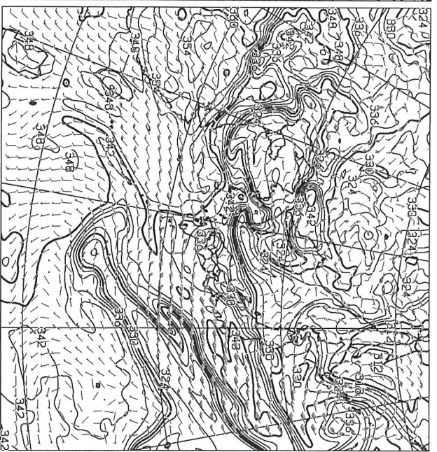
T=24 850hPa: E.P. TEMP(K), WIND(KNOTS) VALID 011200UTC
